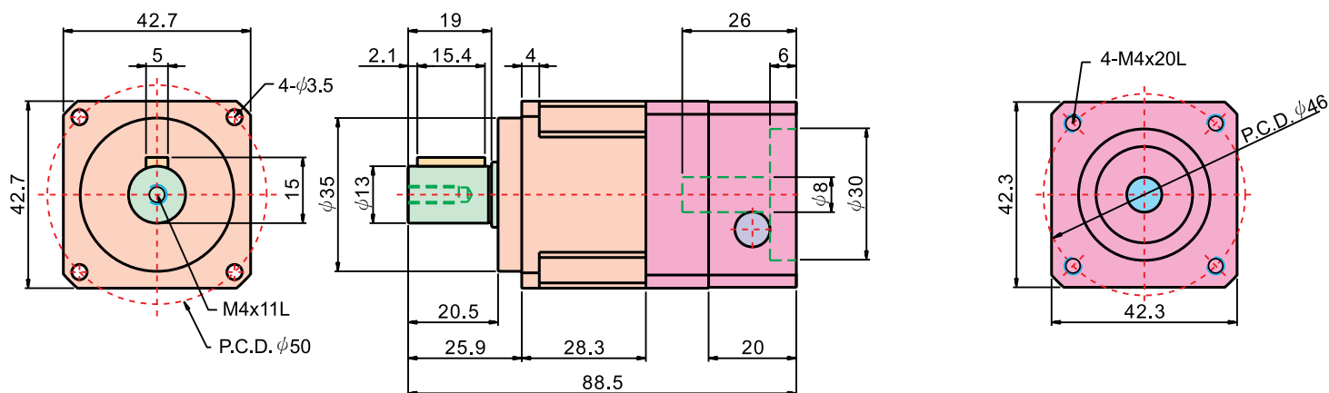
(A) 單節式減速機
